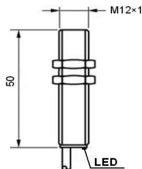
wyjście kablowe / cable output
