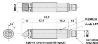
wyjście konektorowe / plug output
