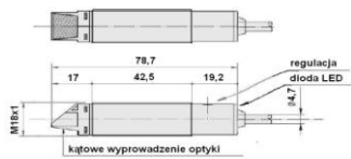
wyjście kablowe / cable output
