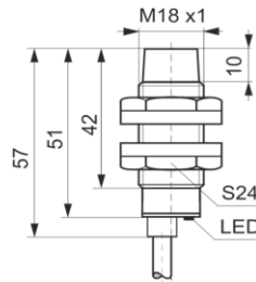
wyjście kablowe / cable output
