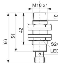
wyjście konektorowe / plug output
