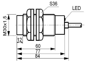
wyjście kablowe / cable output
